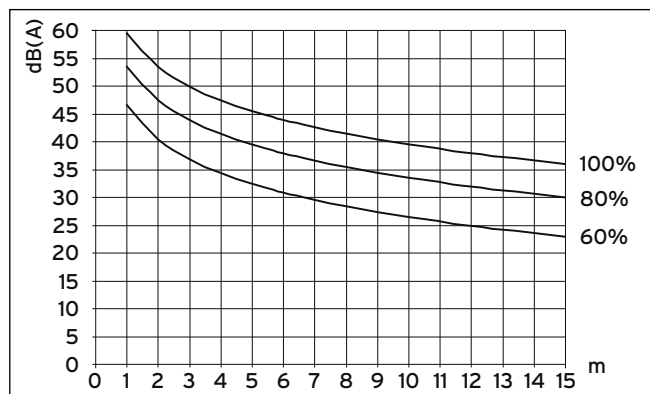
Obr. 6.3 Hladina akustického tlaku venkovní jednotky v dB(A) v závislosti na vzdálenosti a otáčkách ventilátoru pro instalaci VWL 102/3 S na volném prostranství
