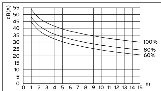
Obr. 6.2 Hladina akustického tlaku venkovní jednotky v dB(A) v závislosti na vzdálenosti a otáčkách ventilátoru pro instalaci VWL 82/3 S na volném prostranství
