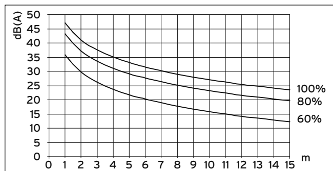
Obr. 6.1 Hladina akustického tlaku venkovní jednotky v dB(A) v závislosti na vzdálenosti a otáčkách ventilátoru pro instalaci VWL 62/3 S na volném prostranství
